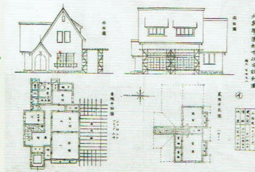
大泉学園都市住宅設計図(大正14年)
